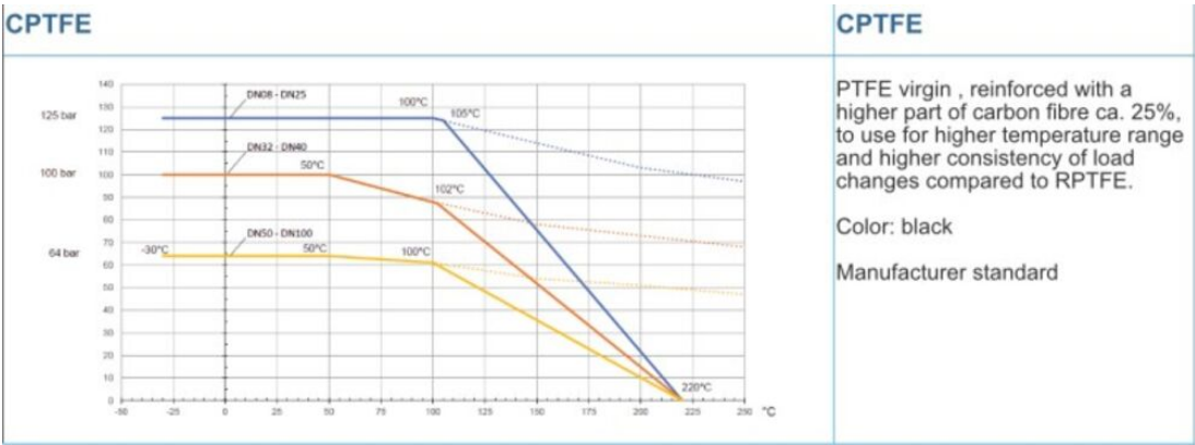
Tryck & temperaturkurva, standardsäten
