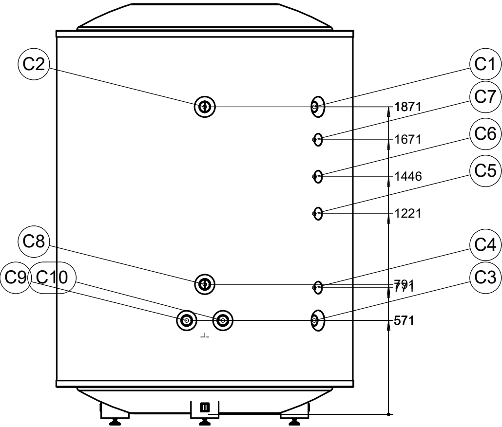
Framsida
