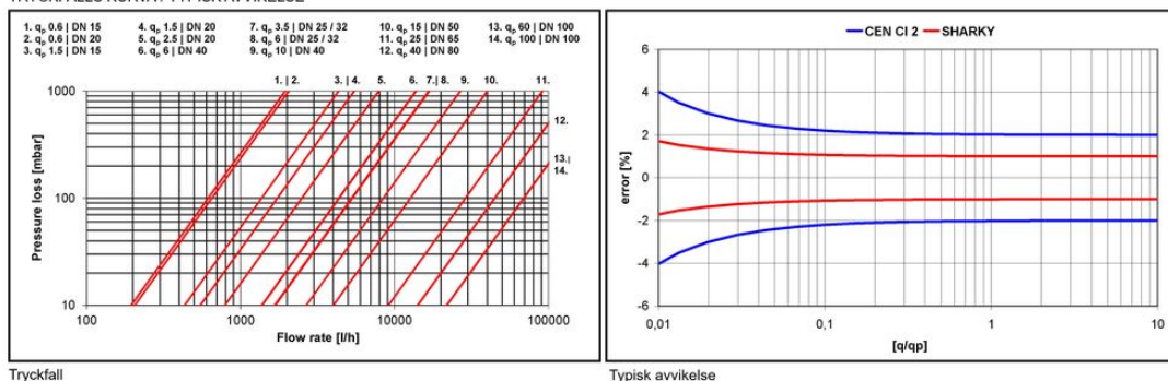
Tryckfall
