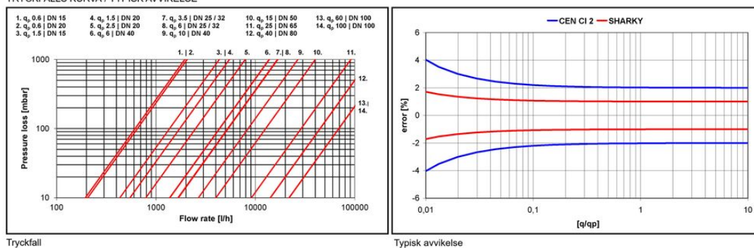
TRYCKFALLS KURVA / TYPISK AVVIKELSE
