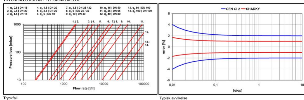
TRYKKFALLS KURVA / TYPISK AVVIKELSE
