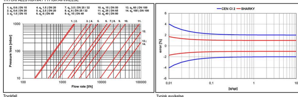
TRYCKFALLS KURVA / TYPISK AVVIKELSE
