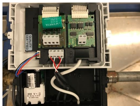
Fig. 7: Anslutningsexempel på temperaturgivare med tvåledar-teknik
