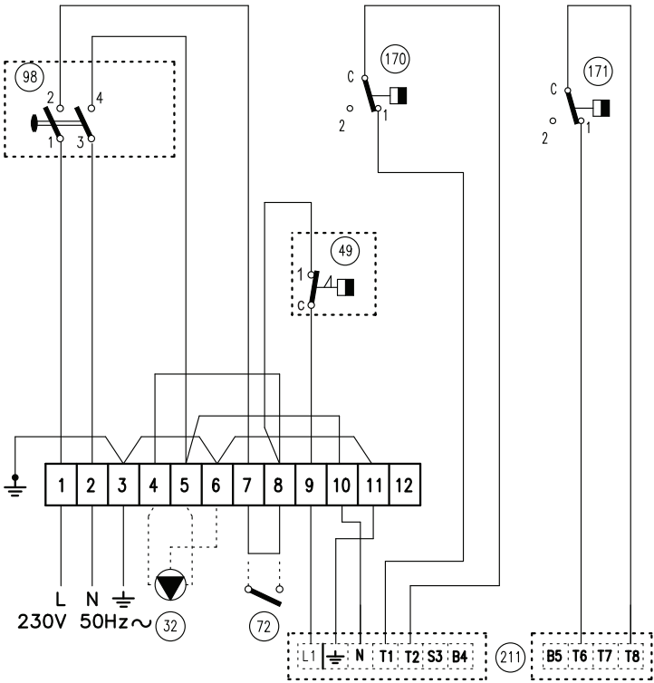
الشكل 10 - مخطط التوصيلات الكهربائية الأساسية ATLAS 95
