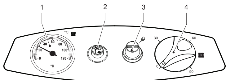
الشكل 1 - لوحة التحكم ومفاتيح التشغيل موديلات ATLAS 32-78
