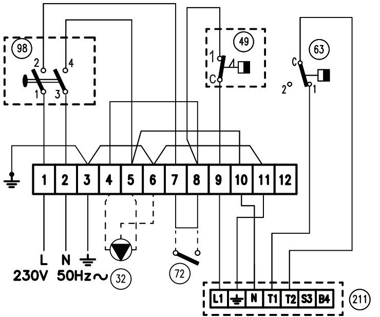
الشكل 8 - مخطط التوصيلات الكهربائية الأساسية ATLAS 32-78
