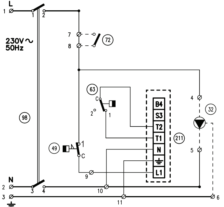
الشكل 7 - مخطط التوصيلات الكهربائية الأساسية ATLAS 32-78
