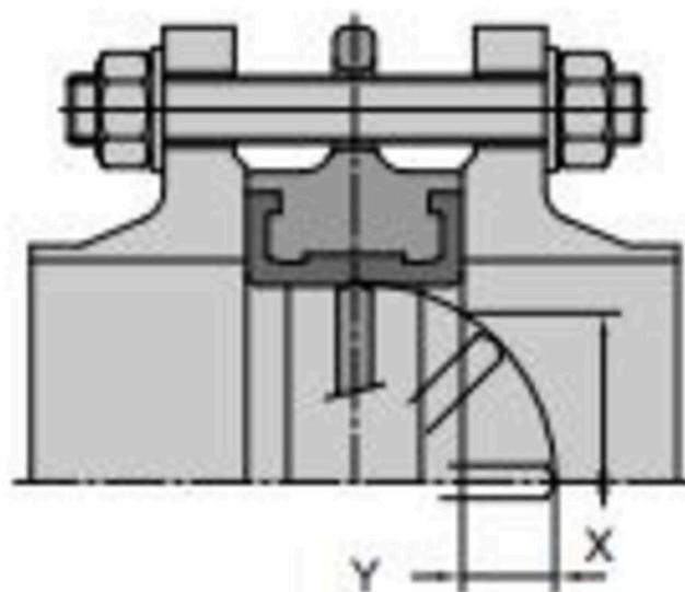
Spjällskivans rörelse
